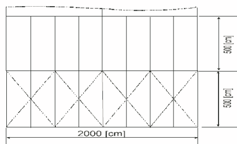
Проекция на покрива
